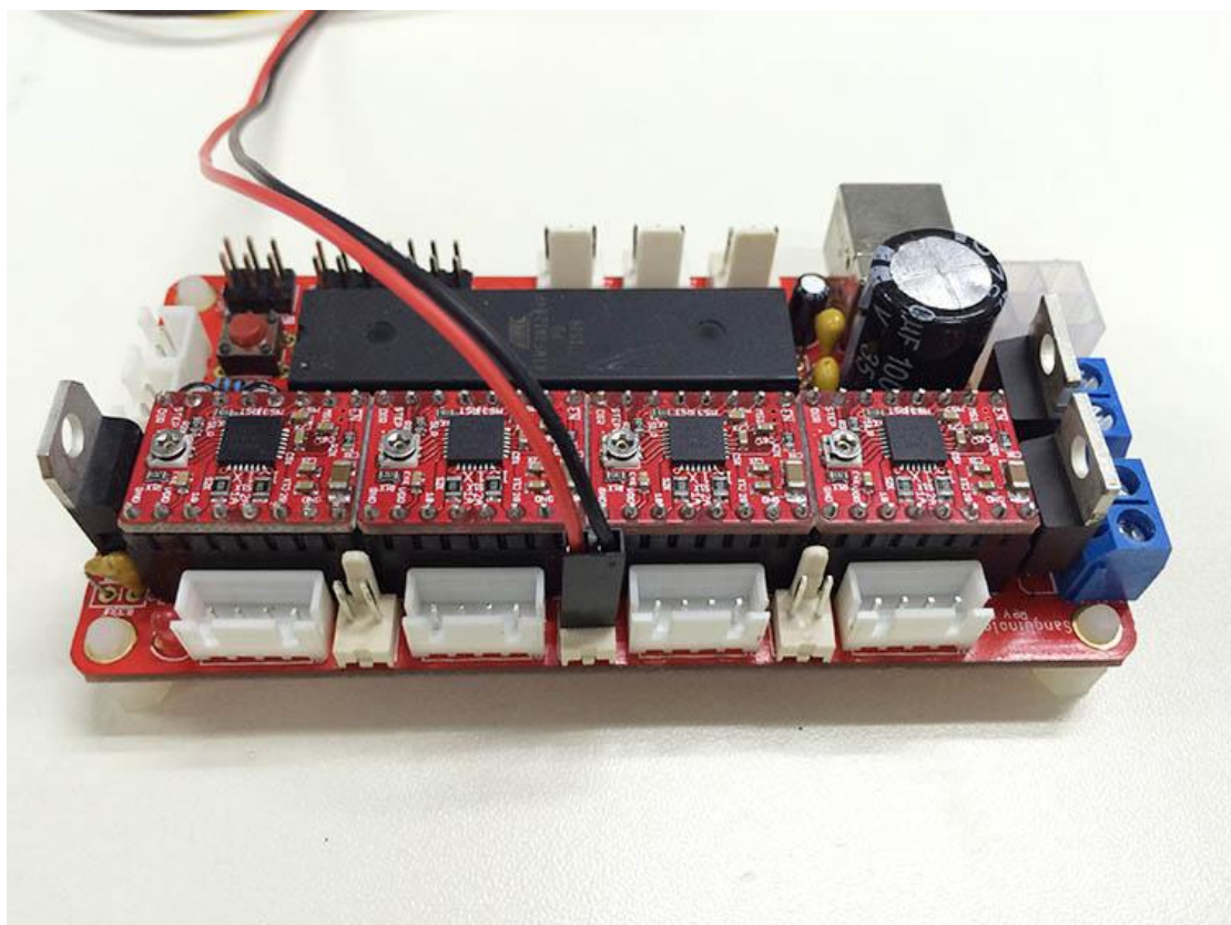
2) Connect fan for extruder.
